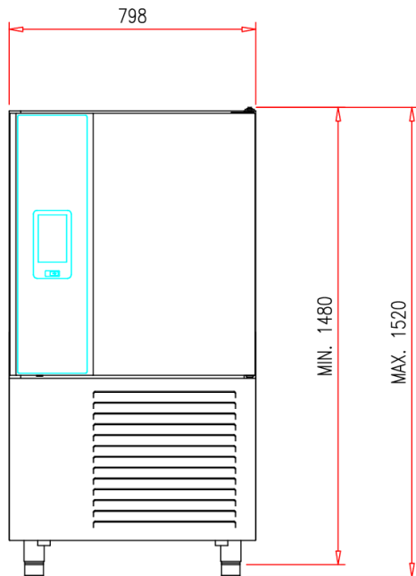
Vorderansicht
