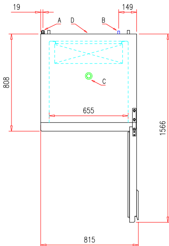
Obenansicht
